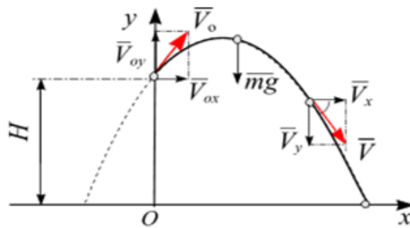
Рисунок 5 – Траектория свободного падения тела с высоты
