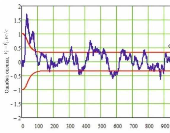
Рисунок 2 – Ошибка оценки скорости изменения времени задержки
